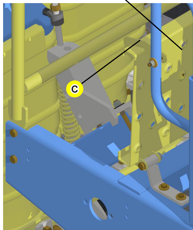
Plataforma na posição para transporte
