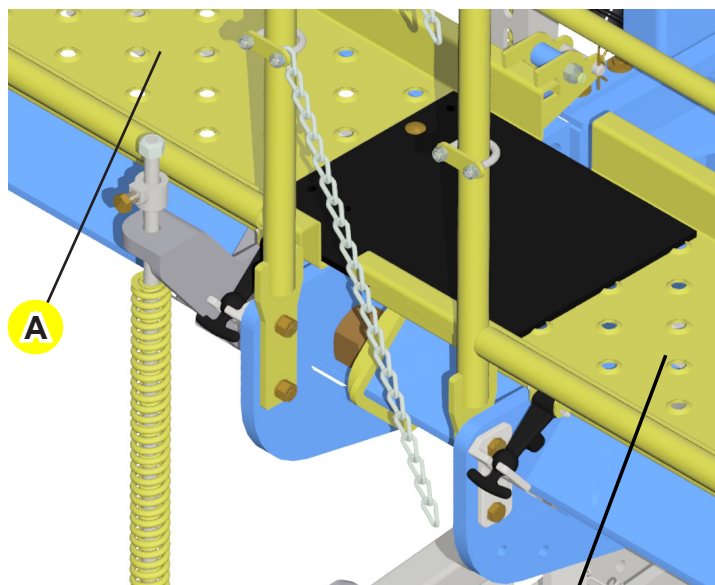
Plataforma na posição para abastecimento
